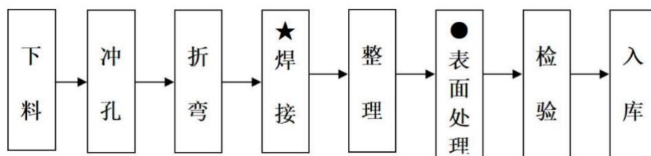
2.3-2 钢制电缆桥架工艺流程图
