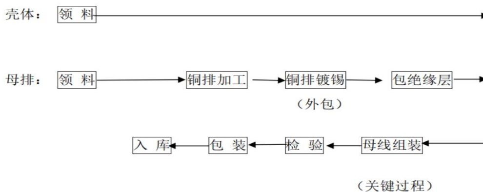
2.3-1 母线槽工艺流程图：
