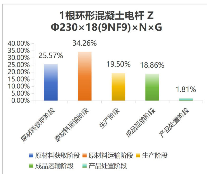
图 5.2-2 一根环形混凝土电杆【ZΦ230×18(9NF9)×N×G】
