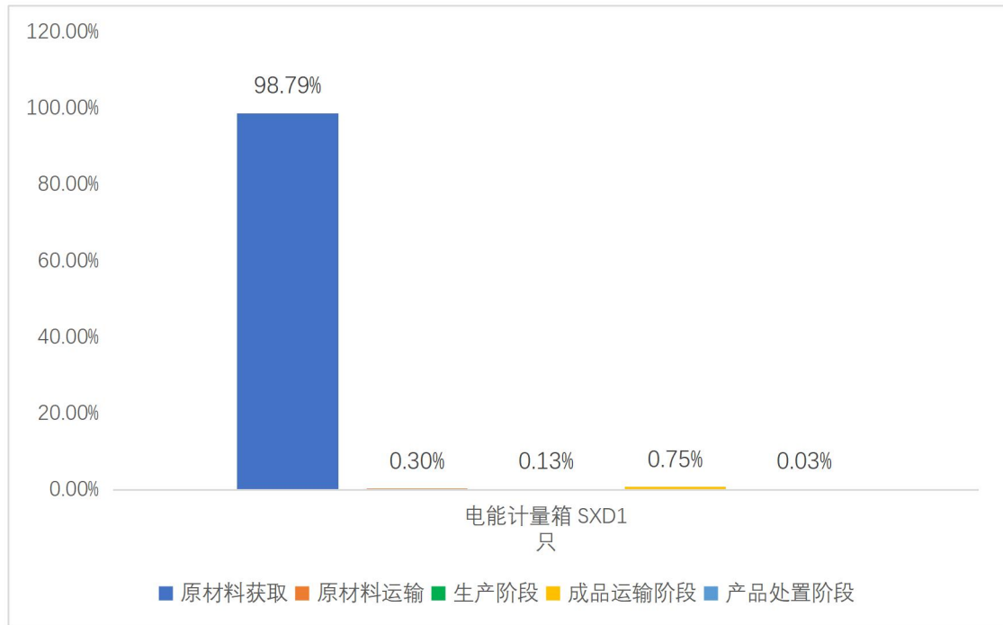
图 5.2-2 电能计量箱 SXD1 生命周期阶段碳排放分布图
