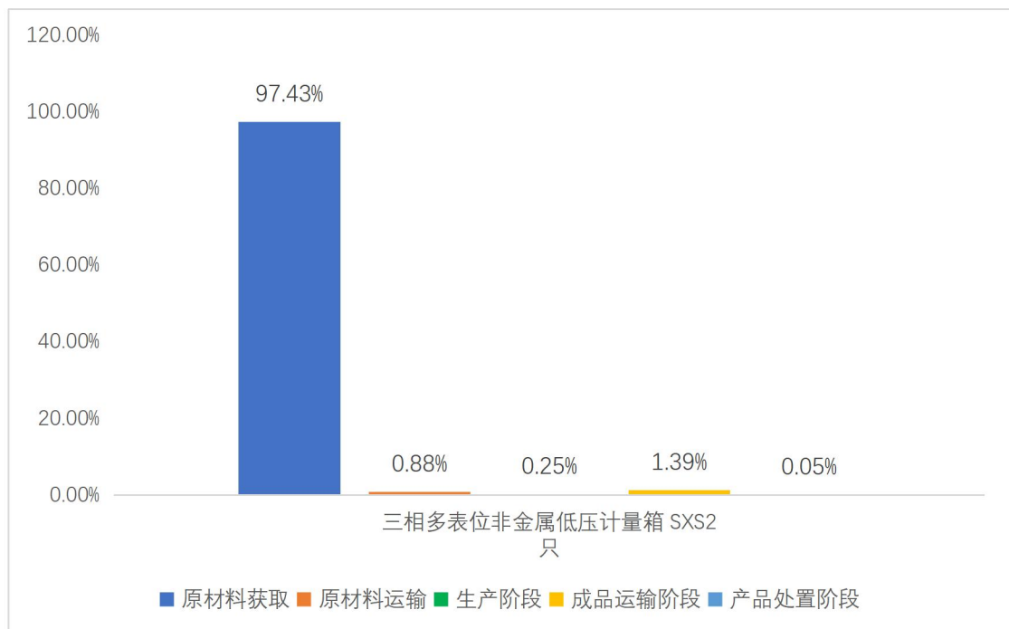
图 5.2-2 三相多表位非金属低压计量箱 SXS2 生命周期阶段碳排放分布图
