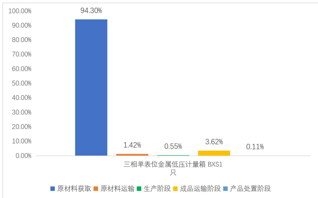
图 5.2-2 三相单表位金属低压计量箱 BXS1 生命周期阶段碳排放分布图
