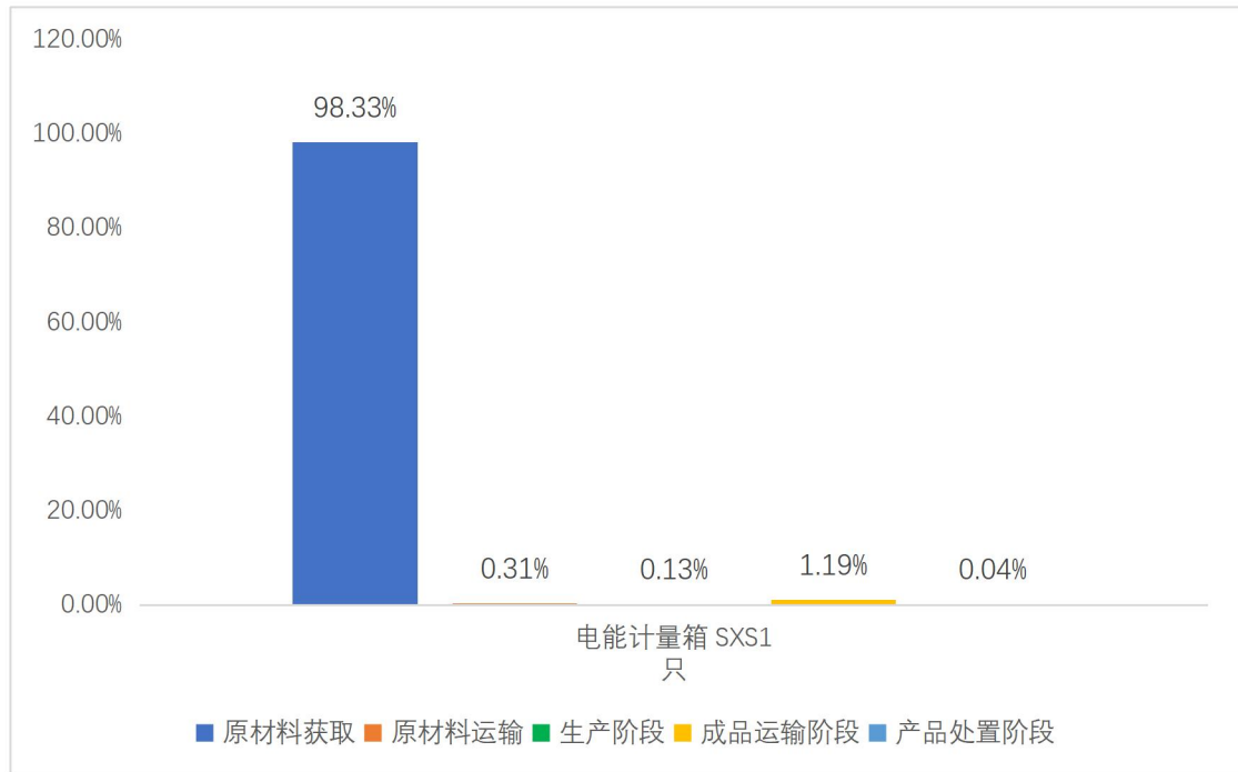
图 5.2-2 电能计量箱 SXS1 生命周期阶段碳排放分布图
