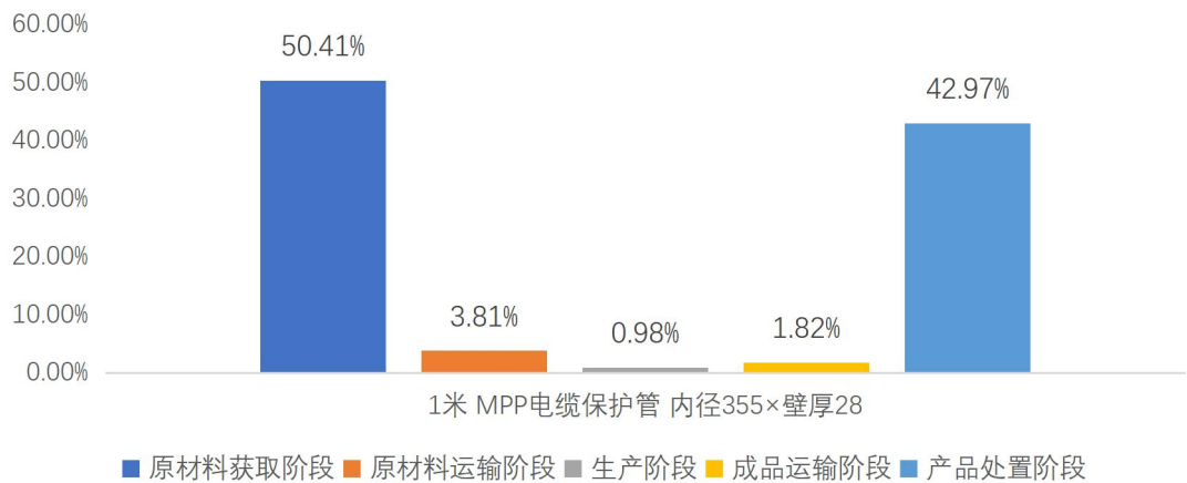
图 5.2-2 MPP 电缆保护管内径 355×壁厚 28 生命周期阶段碳排放分布图
