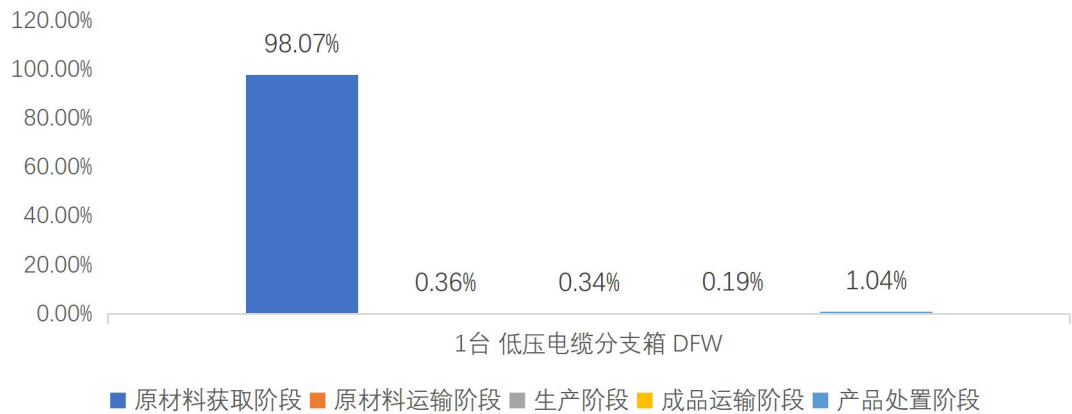
图 5.2-2 低压电缆分支箱 DFW 生命周期阶段碳排放分布图
