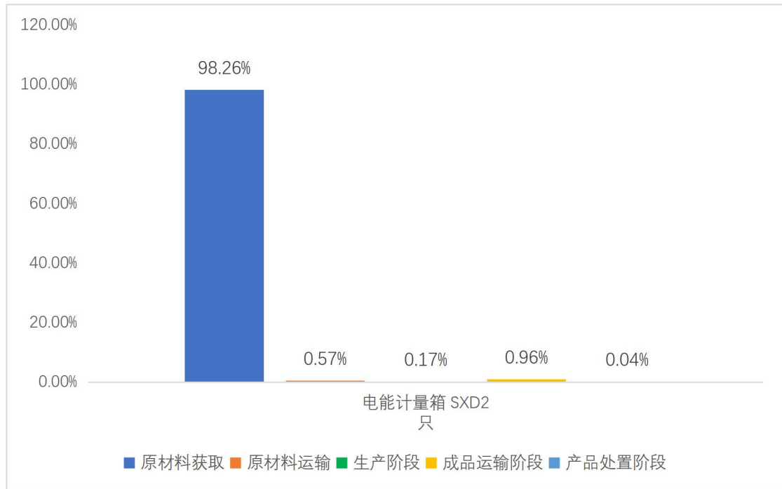
图 5.2-2 电能计量箱 SXD2 生命周期阶段碳排放分布图
