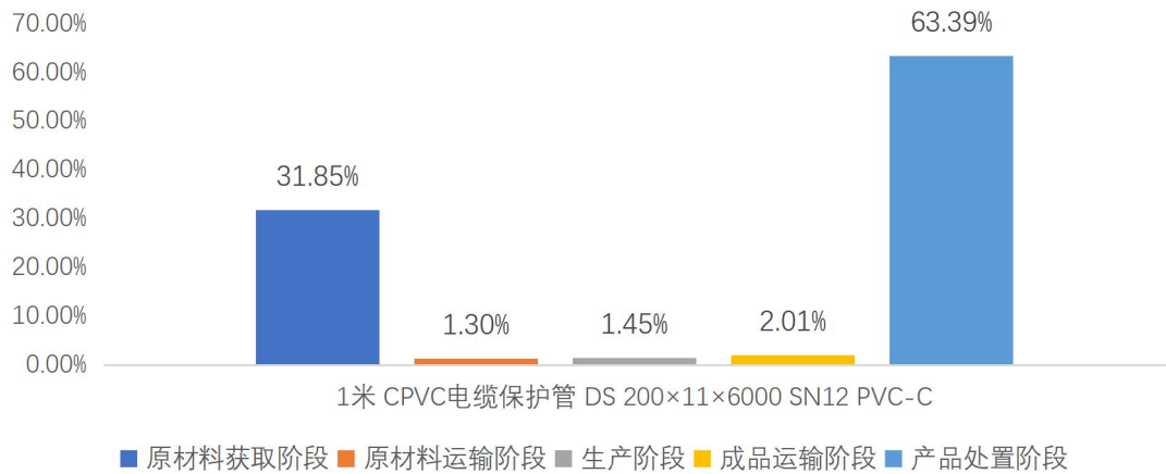
图 5.2-2 CPVC 电缆保护管 DS 200×11×6000 SN12 PVC-C 生命周期阶段碳排放分布图
