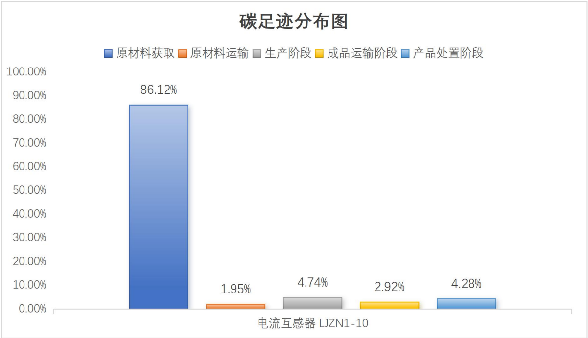
图 5.2.1-2 产品生命周期阶段碳排放分布图
