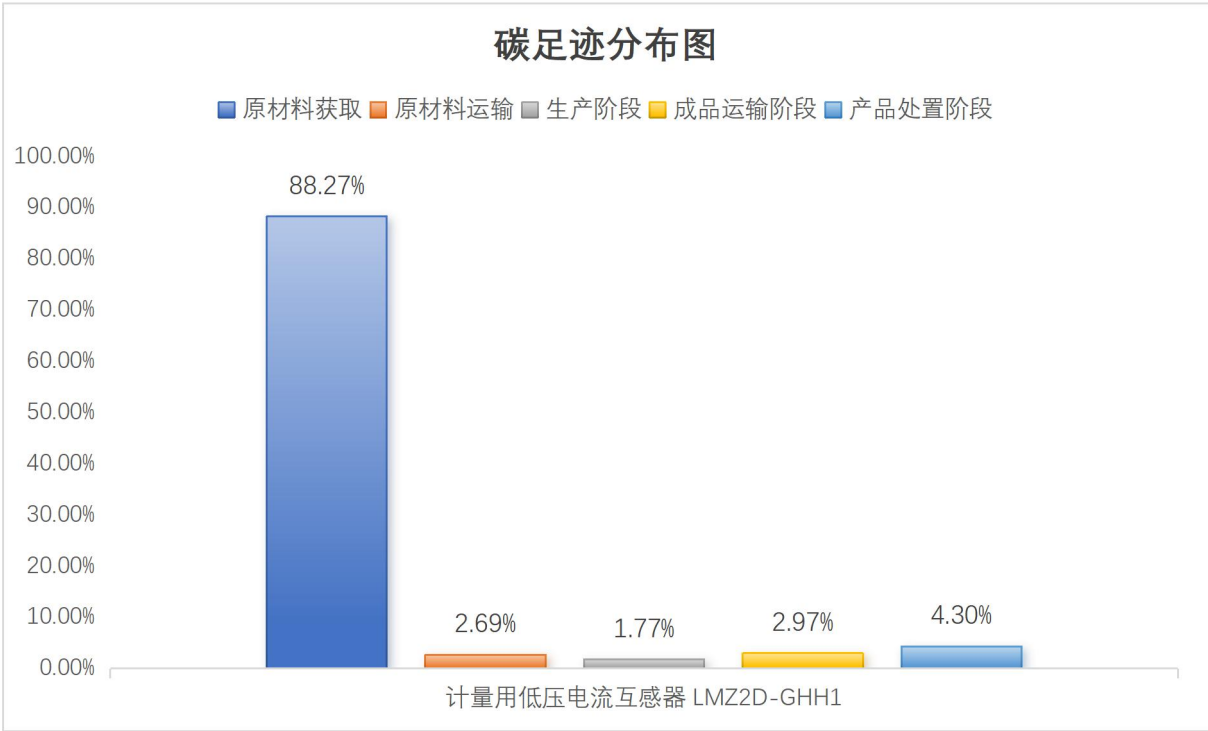
图 5.2.1-2 产品生命周期阶段碳排放分布图
