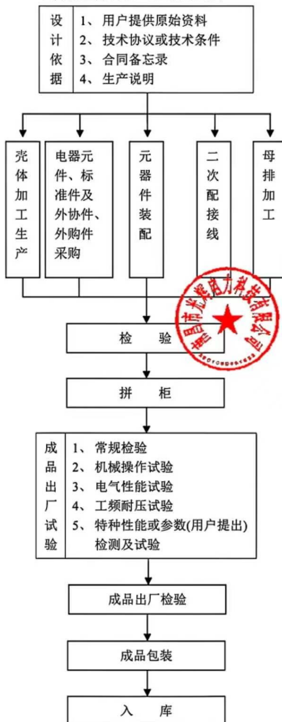
高低压成套工艺流程图
