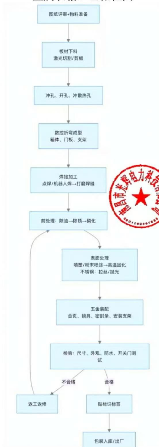
金属表箱工艺流程图
