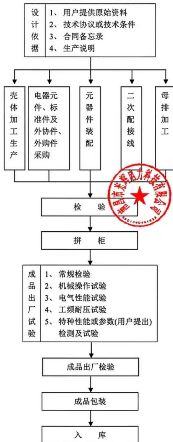
高低压成套工艺流程图
