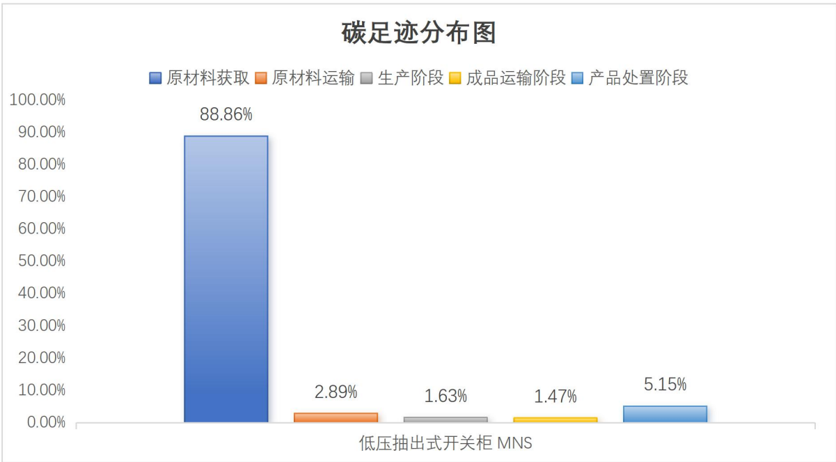
图 5.2.1-2 产品生命周期阶段碳排放分布图
