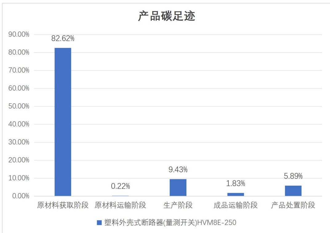
图 5.2.2 塑料外壳式断路器(量测开关) (HVM8E-250) 生命周期阶段碳排放分布图
