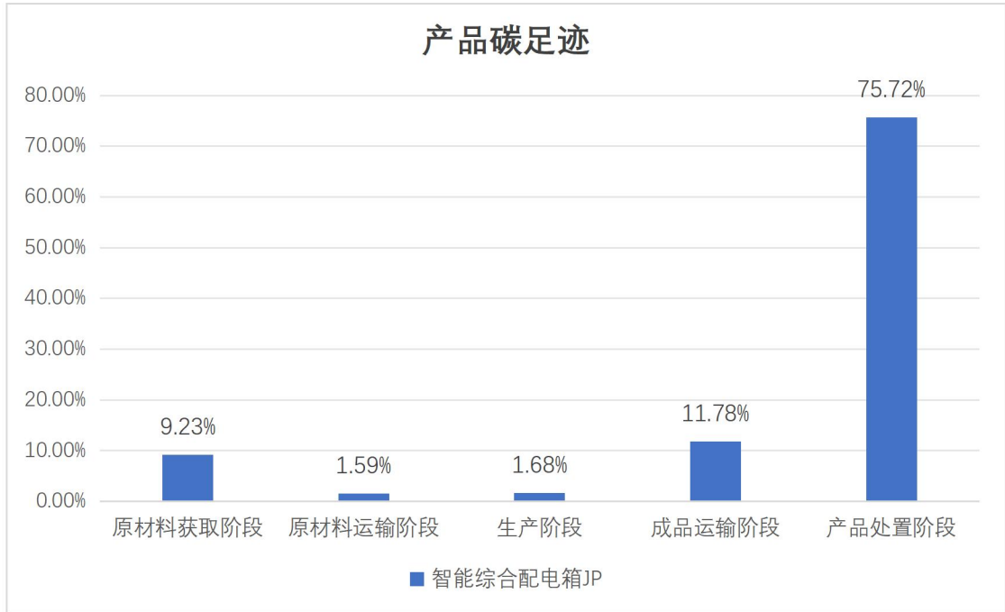
图 5. 2. 2 智能综合配电箱（JP）生命周期阶段碳排放分布图
