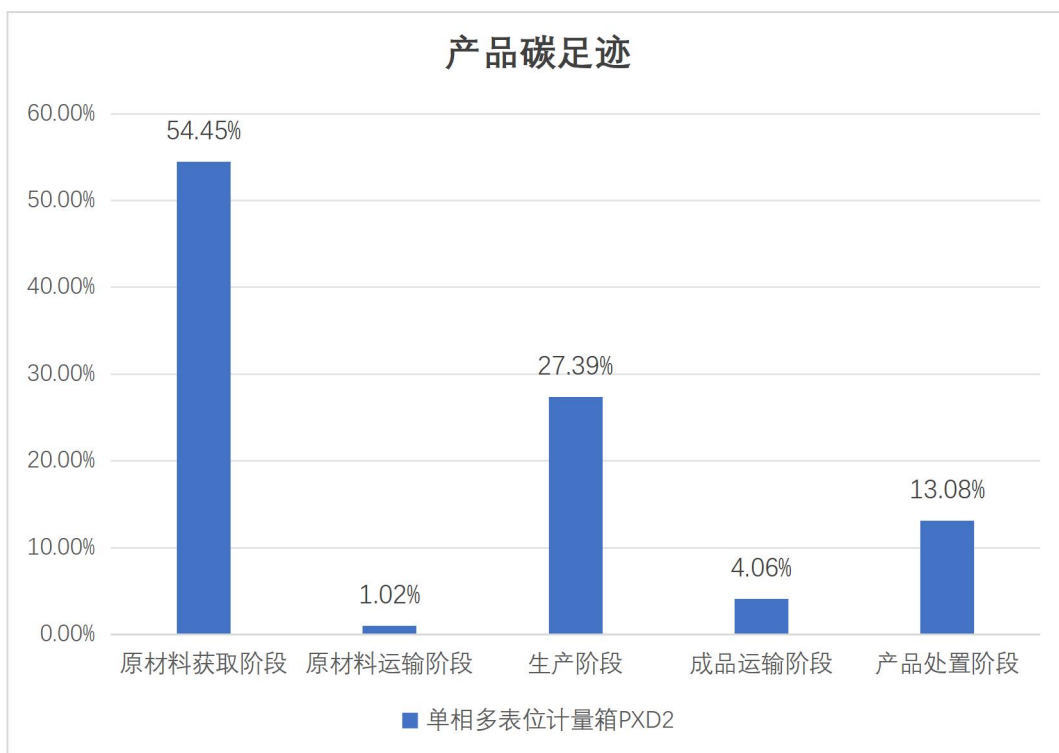
图 5.2.2 单相多表位计量箱（PXD2）生命周期阶段碳排放分布图
