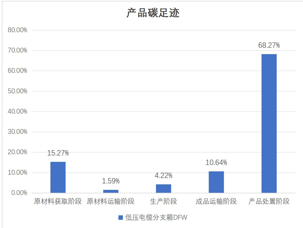
图 5.2.2 低压电缆分支箱（DFW）生命周期阶段碳排放分布图
