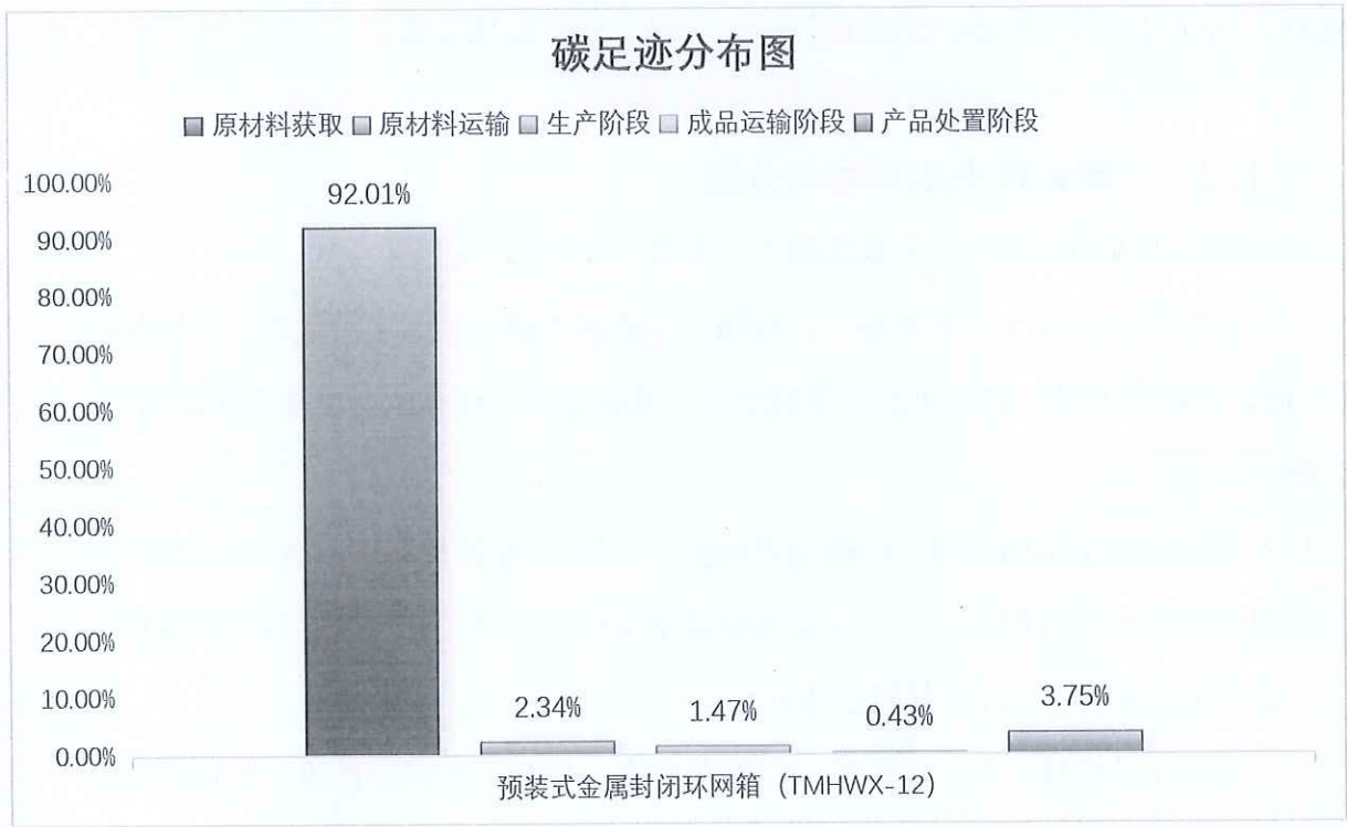
图 5.2.1-2 产品生命周期阶段碳排放分布图
