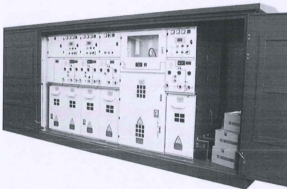
预装式金属封闭环网箱 XGW-12(630-20)
