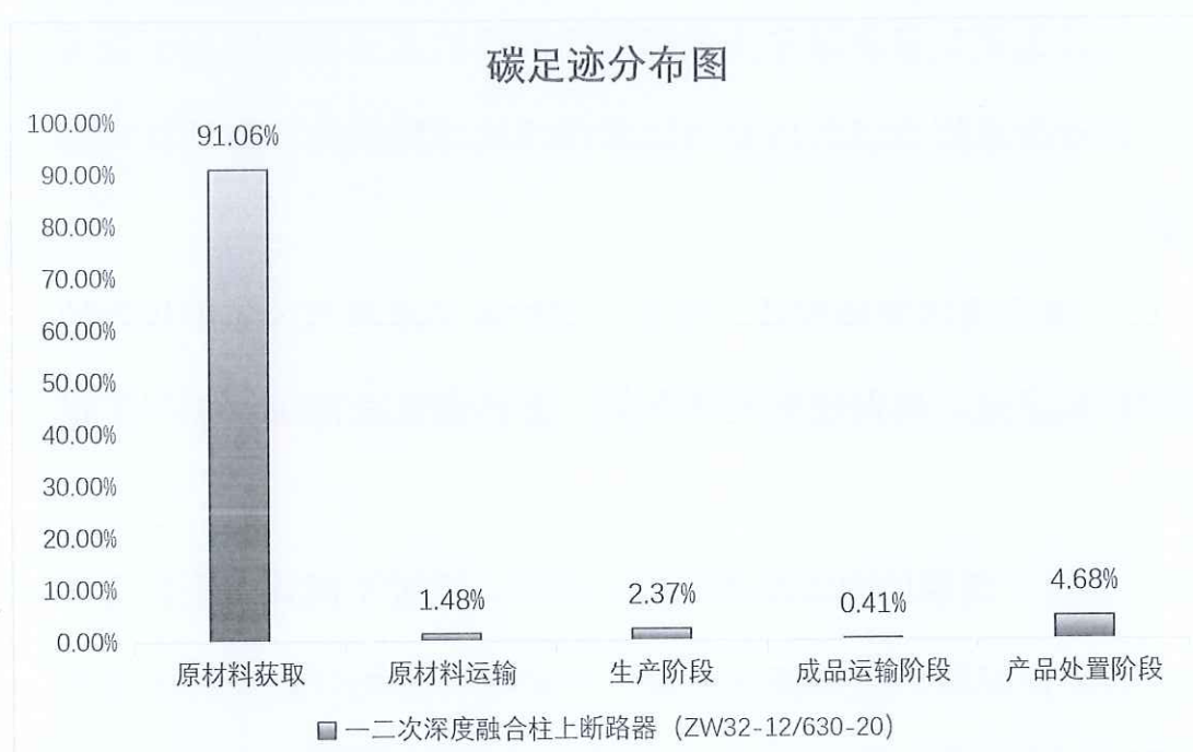
图 5.2.1.2 一二次深度融合柱上断路器（ZW32-12/630-20）生命周期阶段碳排放分布图
