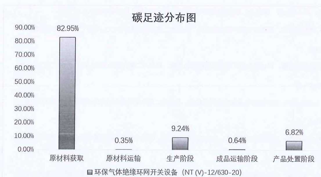
图 5.2.1.2 环保气体绝缘环网开关设备 (NT (V)-12/630-20) 生命周期阶段碳排放分布图
