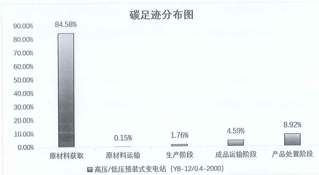
图 5.2.1.2 高压/低压预装式变电站（YB-12/0.4-2000）生命周期阶段碳排放分布图
