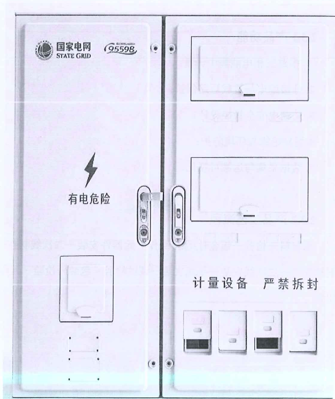
三相多表位非金属低压计量箱 (PXS2)
