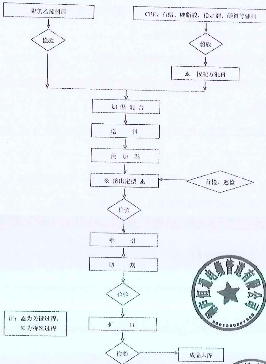
氯化聚氯乙烯塑料电缆管道生产工艺流程图 ( QZ751-02-2012 )
