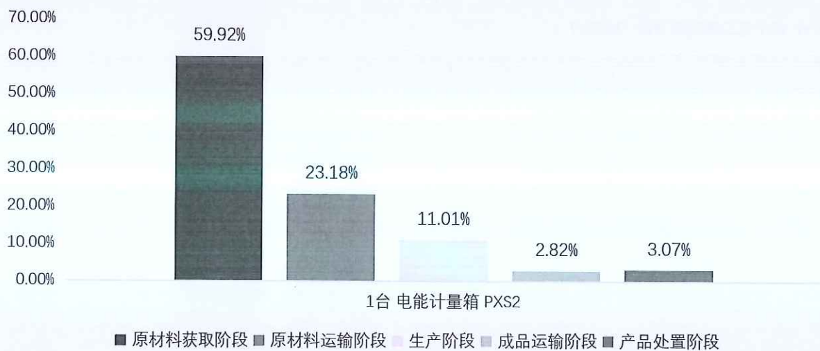
图 5.2.1-2 产品生命周期阶段碳排放分布图
