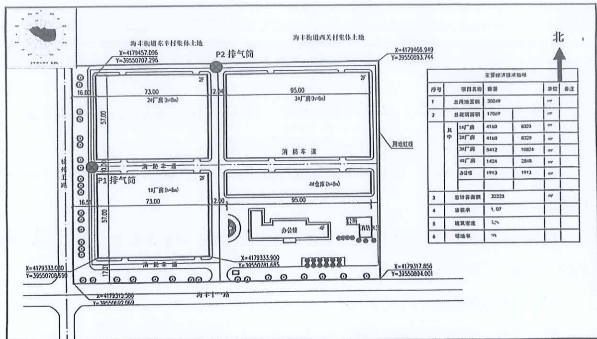
附图3 项目厂区总平布置图 比例尺: 1:1000
