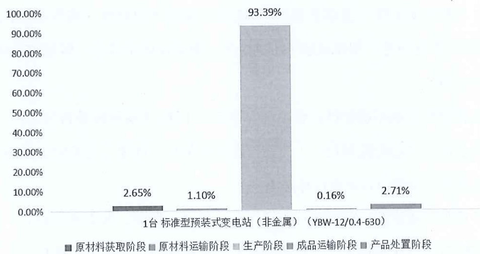
图 5.2.1-2 产品生命周期阶段碳排放分布图
