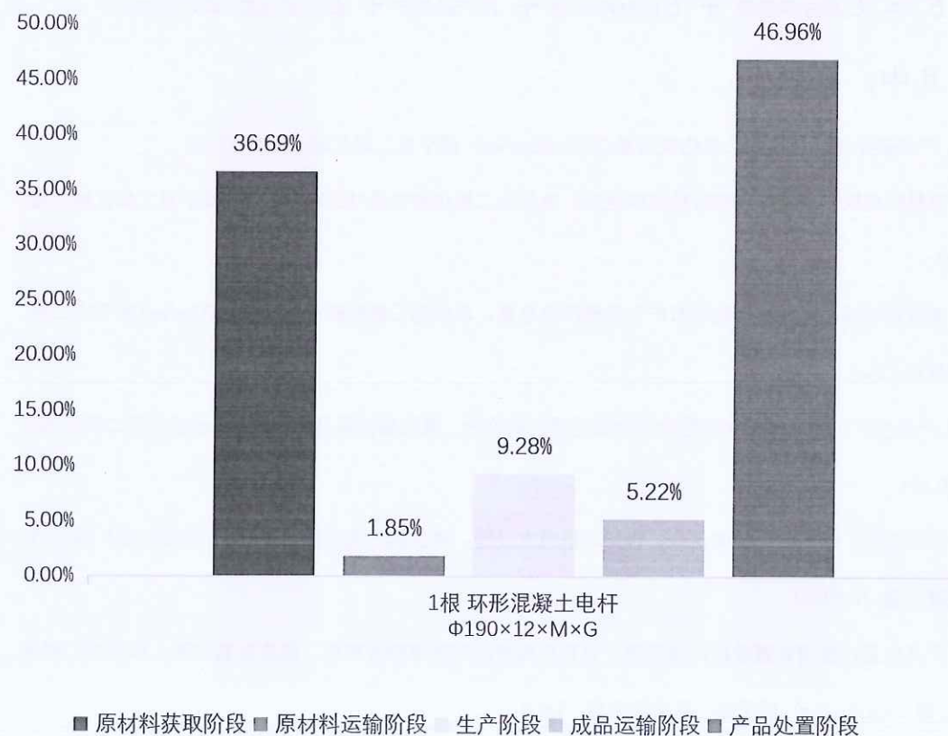
图 5.2-2 生命周期阶段碳排放分布图
