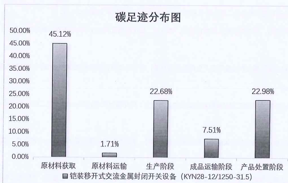
图 5.2.1.2 铠装移开式交流金属封闭开关设备（KYN28-12/1250-31.5）生命周期阶段碳排放分布图
