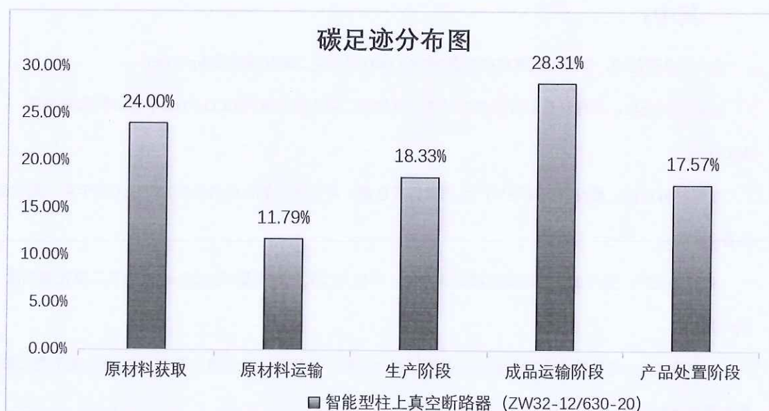
图 5.2.1.2 智能型柱上真空断路器（ZW32-12/630-20）生命周期阶段碳排放分布图
