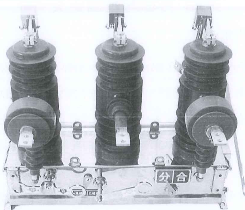
智能型柱上真空断路器 (ZW32-12/630-20)
