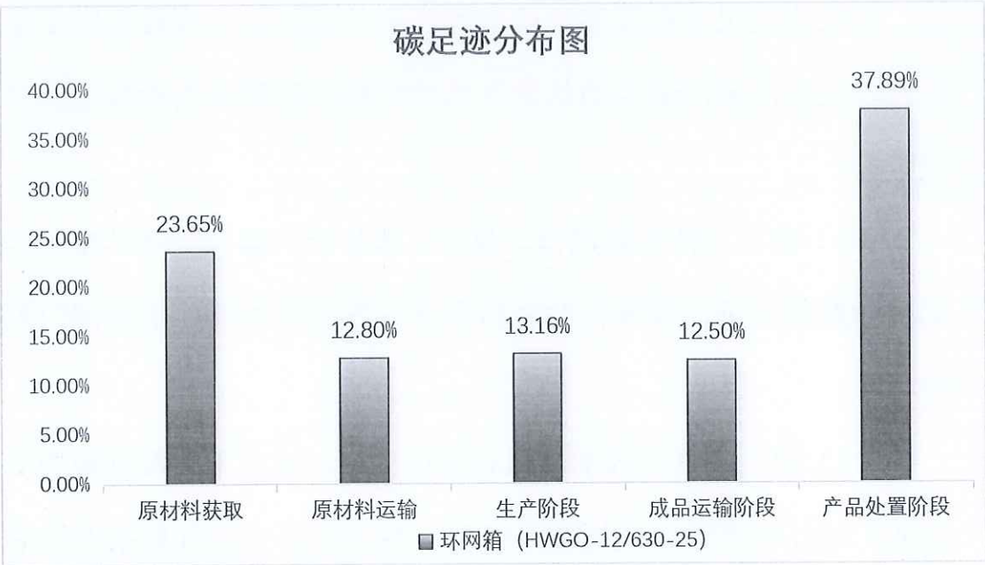
图 5.2.1.2 环网箱（HWGO-12/630-25）生命周期阶段碳排放分布图
