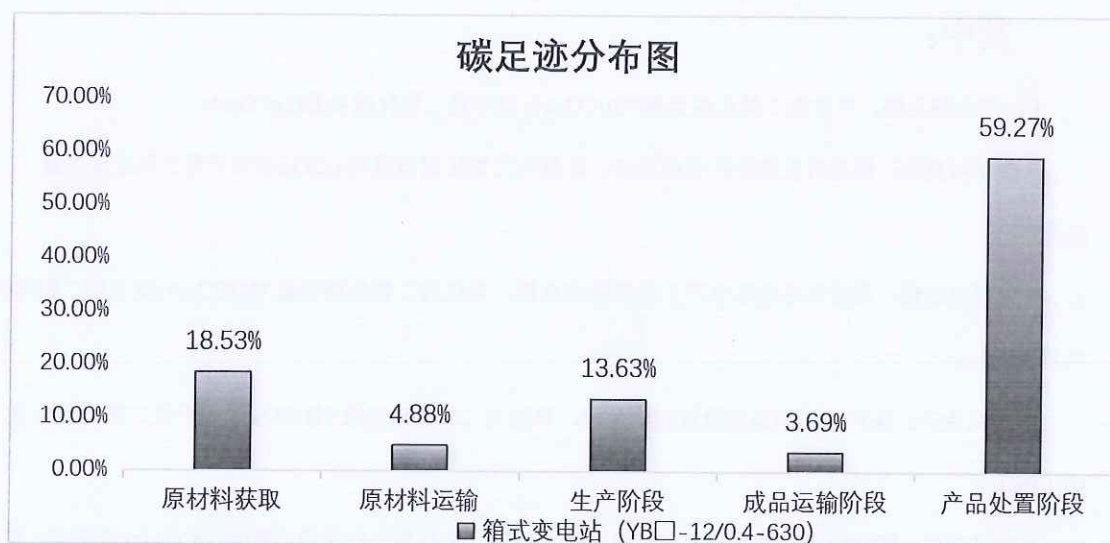
图 5. 2. 1. 2 箱式变电站 (YB□-12/0. 4-630) 生命周期阶段碳排放分布图
