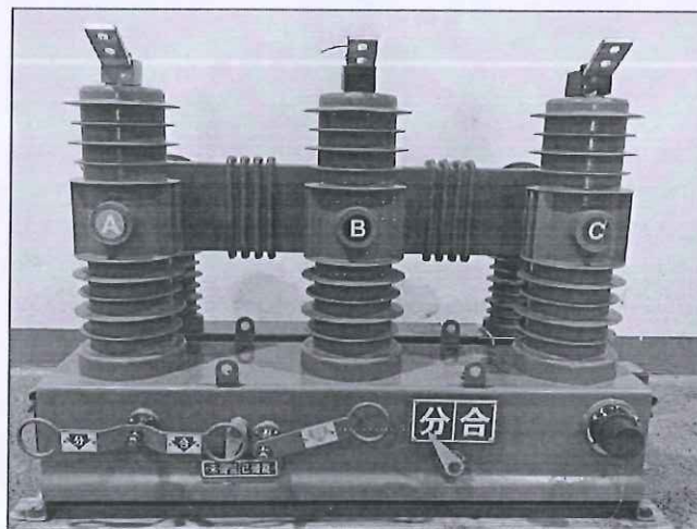
户外高压交流柱上真空断路器 ZW32-12/T630-25
