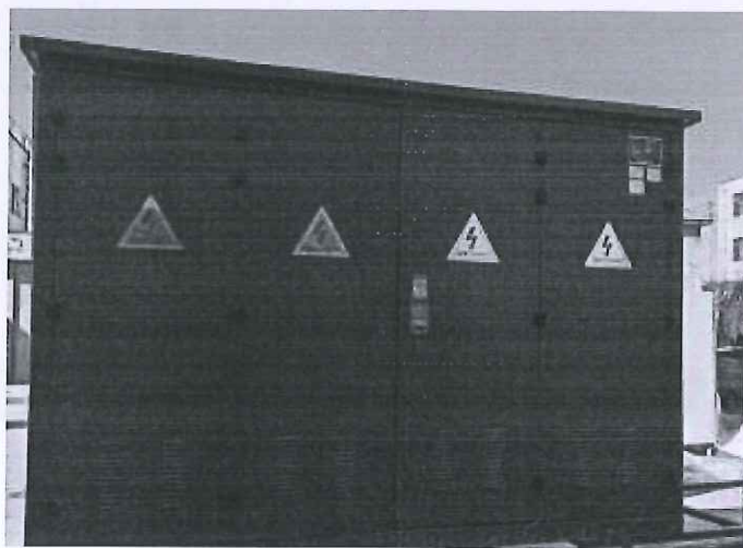
预装式金属封闭环网箱 RZXGW-12
