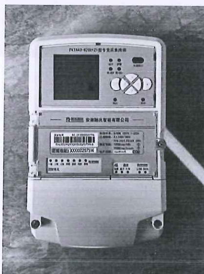
专变采集终端 III 型 FKTA43-RZ001Z1
