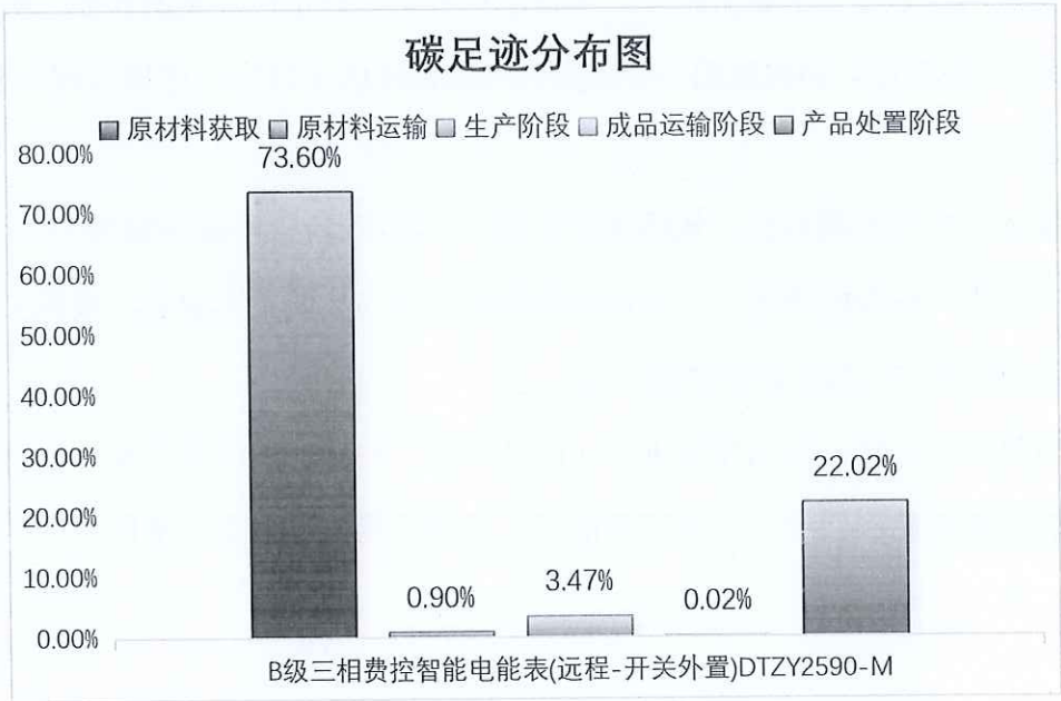
图 5.2.2 产品生命周期阶段碳排放分布图
