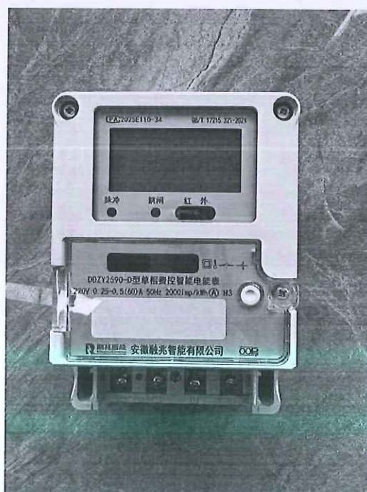
A 级单相费控智能电能表(远程-开关外置) DDZY2590-M
