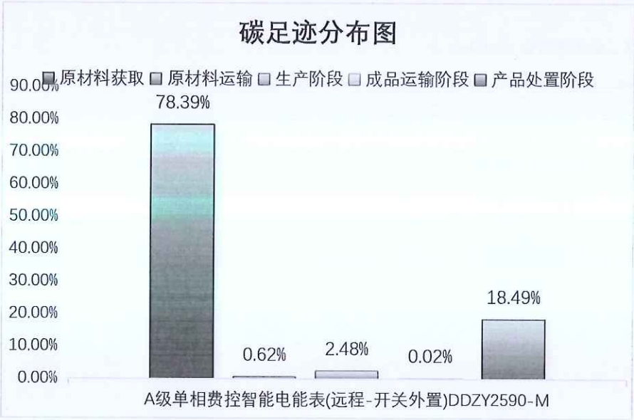
图 5.2.2 产品生命周期阶段碳排放分布图
