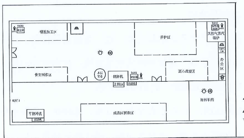
附图3 项目平面布置图
