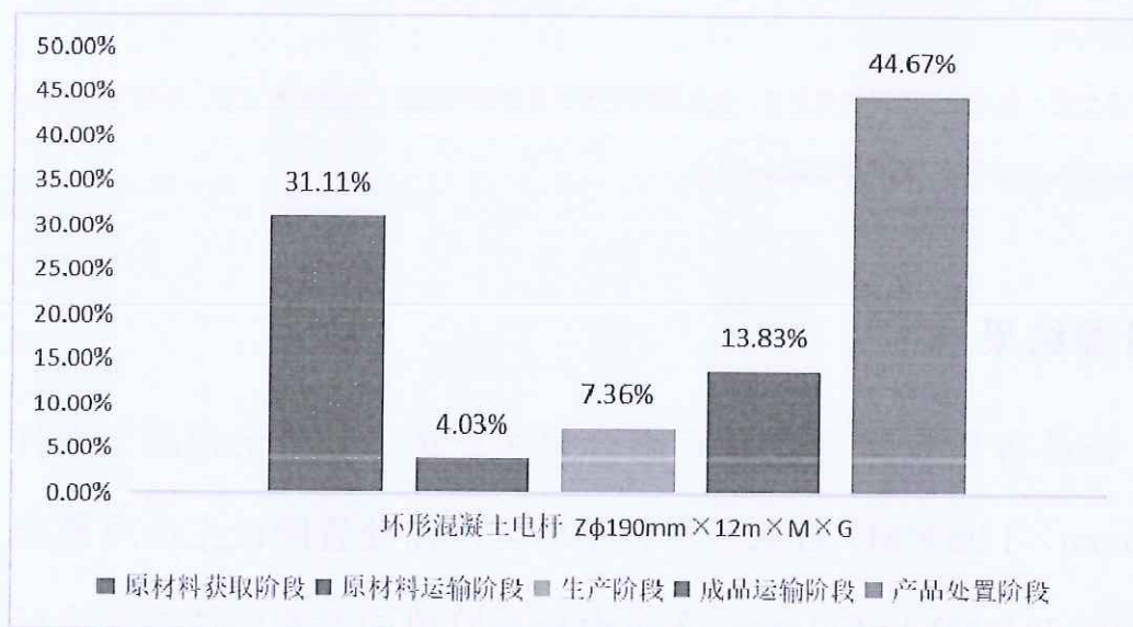
图 5.2.2 环形混凝土电杆 \Phi 190\text{mm} \times 12\text{m} \times \text{M} \times \text{G} (生命周期阶段碳排放分布图)
