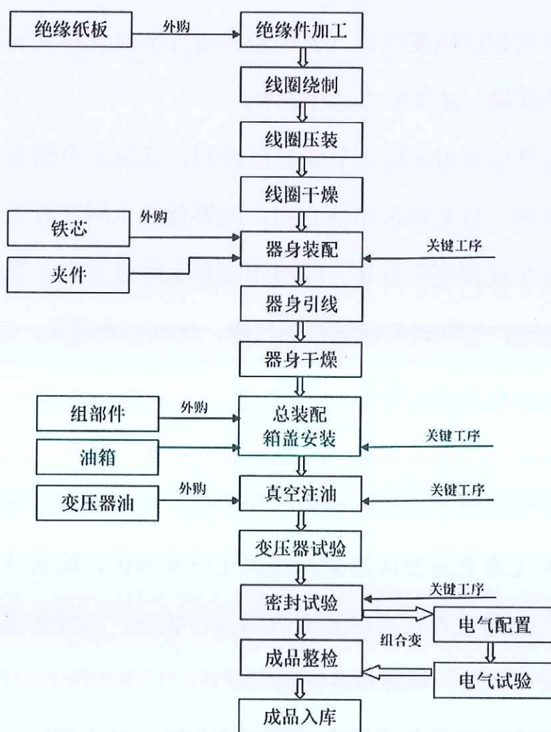
油浸式变压器工艺流程图
