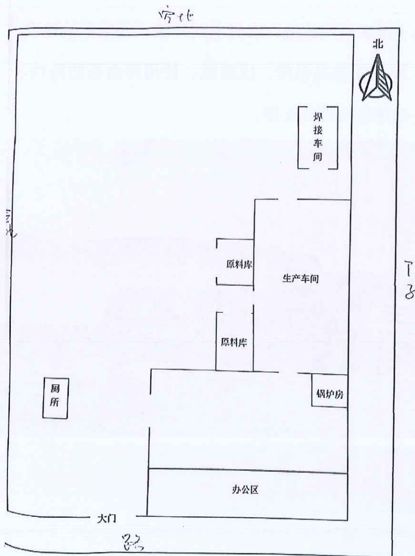
附图3 建设项目平面布置图
