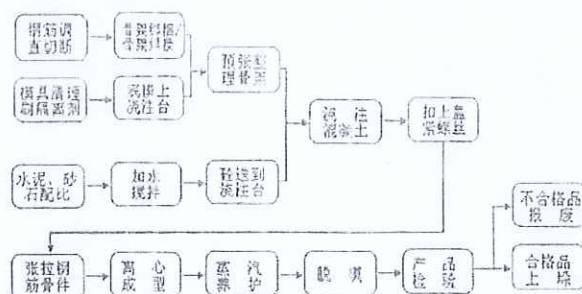
1. 环形混凝土电杆工艺流程图
