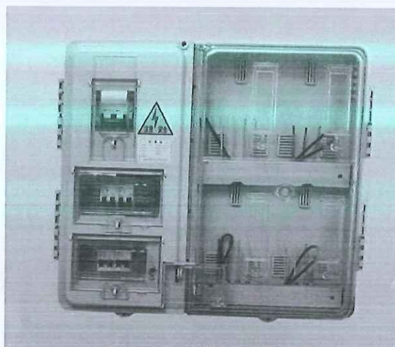
单相多表位非金属低压计量箱-过盈配合接插件 PXD2
