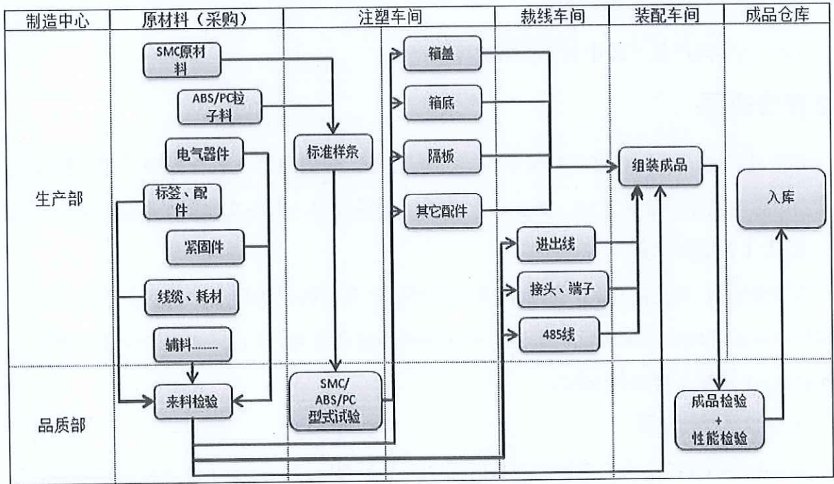
非金属表箱流程图
