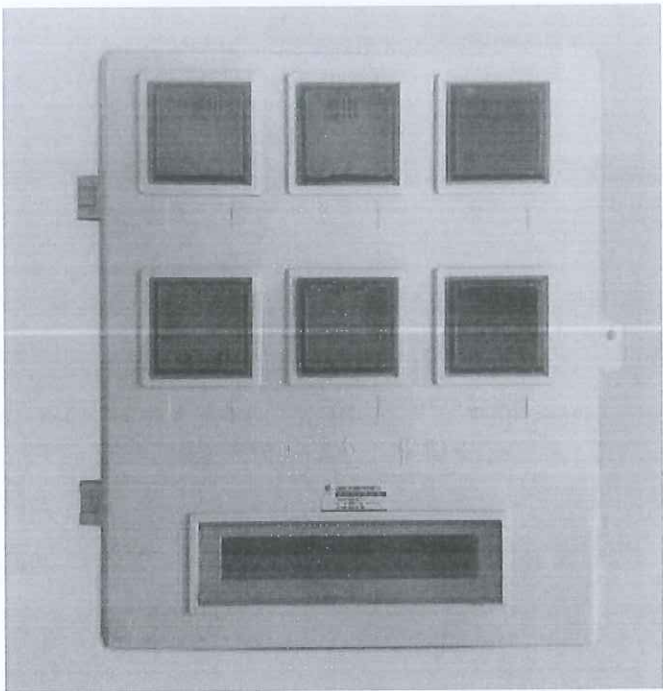
单相多表位非金属低压计量箱-过盈配合接插件 SXD2
