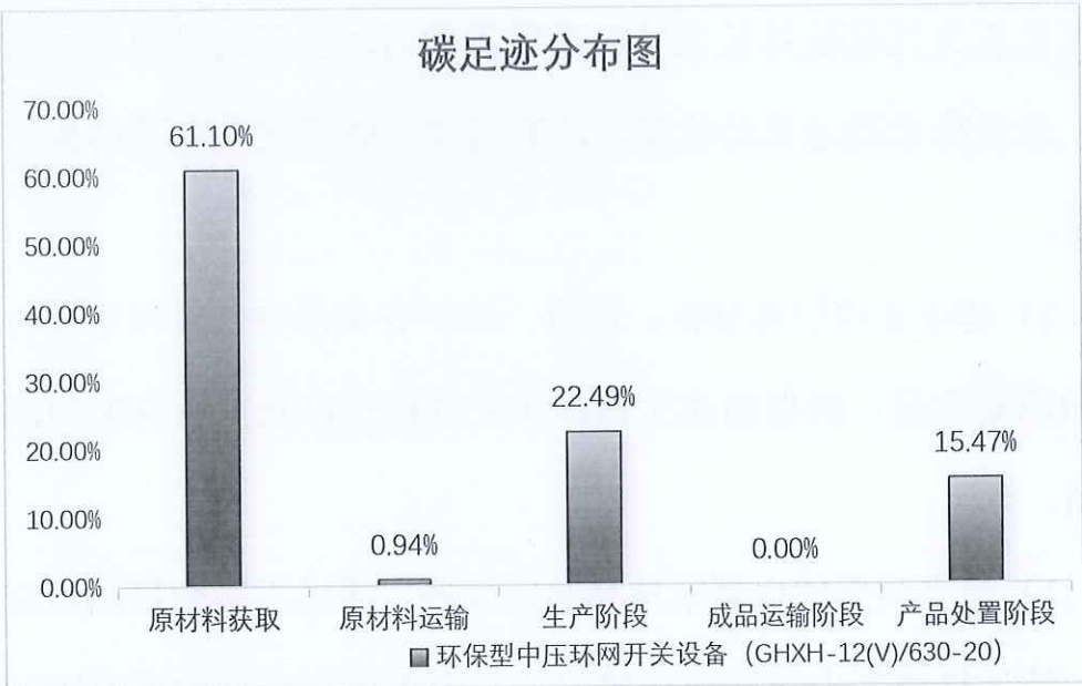
图 5.2.1.2 环保型中压环网开关设备 (GHXH-12(V)/630-20) 生命周期阶段碳排放分布图
