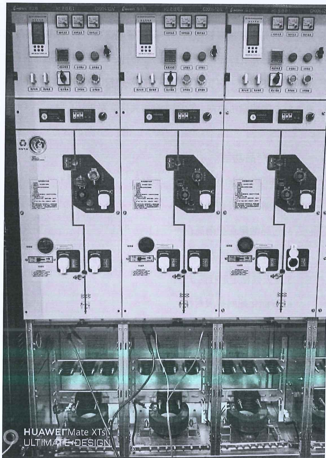
环保型中压环网开关设备 (GHXH-12(V)/630-20)
