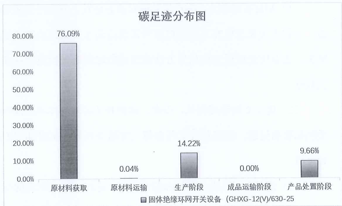
图 5.2.1.2 固体绝缘环网开关设备 (GHXG-12(V)/630-25) 生命周期阶段碳排放分布图
