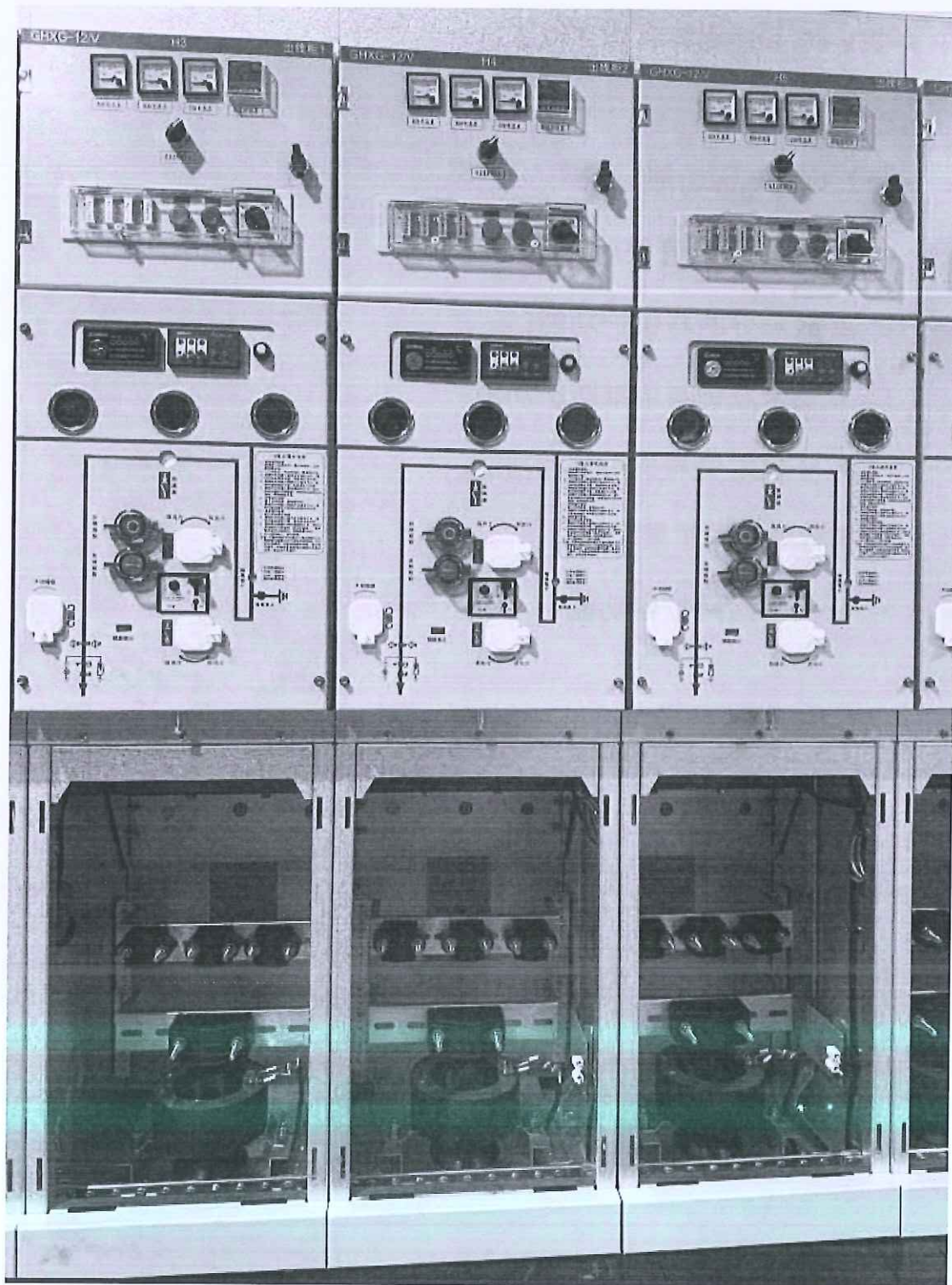
固体绝缘环网开关设备 (GHXG-12(V)/630-25)
