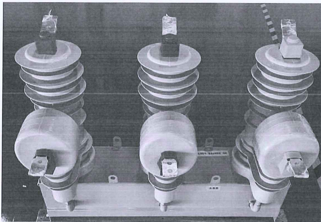
智能户外高压真空断路器 (ZW32-12/T630-25)
