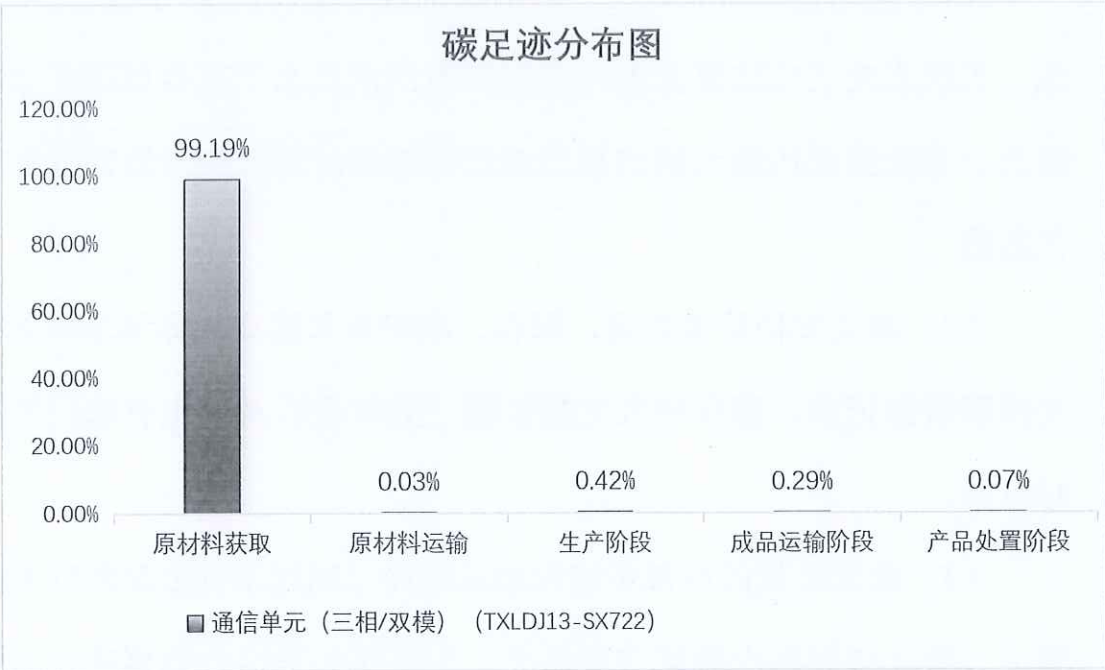
图 5.2.1.2 通信单元（三相/双模）（TXLDJ13-SX722）生命周期阶段碳排放分布图
