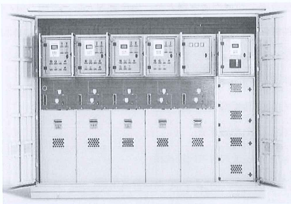
高压环网箱(开闭所) (HHWX-12)
