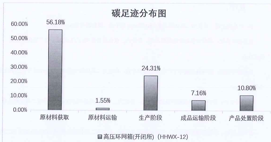
图 5. 2. 1. 2 高压环网箱(开闭所) (HHWX-12) 生命周期阶段碳排放分布图
